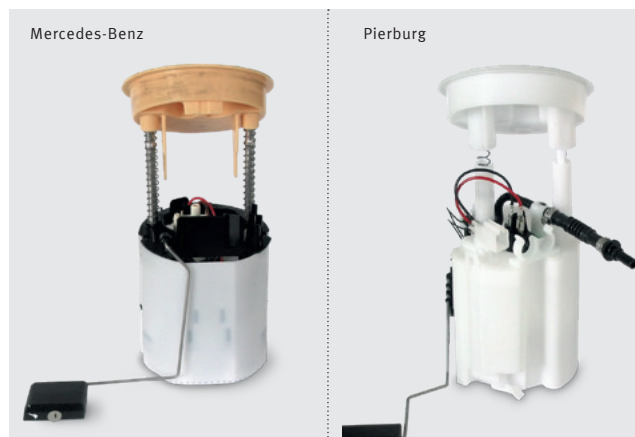
Abb. 1: Kraftstofffördermodule im Vergleich
