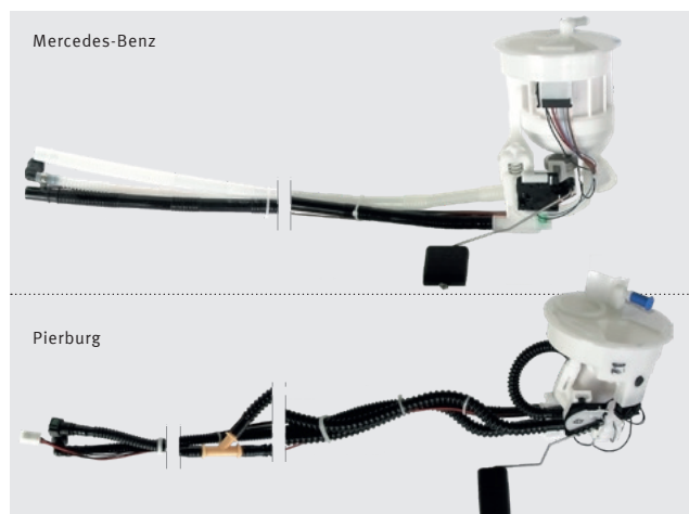
Abb. 2: Tankgebereinheiten im Vergleich
